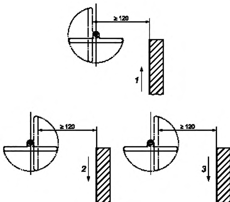
1 – направление движения наклоняющейся льюшки; 2 – направление движения мягкой льюшки; 3 – направление движения жесткой льюшки
