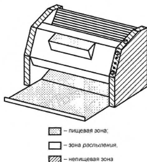
Рисунок 15 — Тестоформирующая машина 1-го типа
