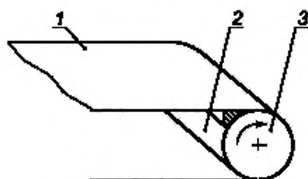
Рисунок 13 — Схема тестоформирующей машины 3-го типа
