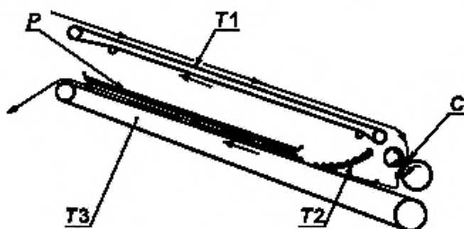
Рисунок 4 — Схема тестоформирующей машины 3-го типа
