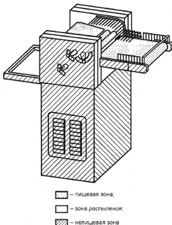
Рисунок 16 — Тестоформирующая машина 2-го типа
