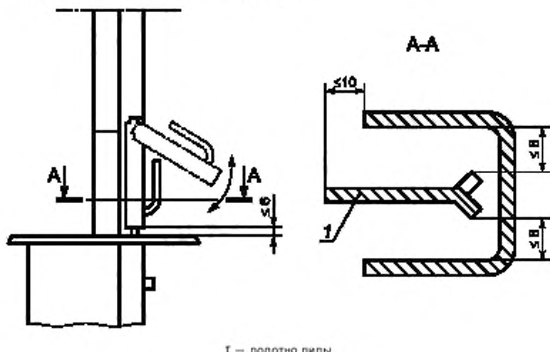
Рисунок 6 — Толкатель продукта
