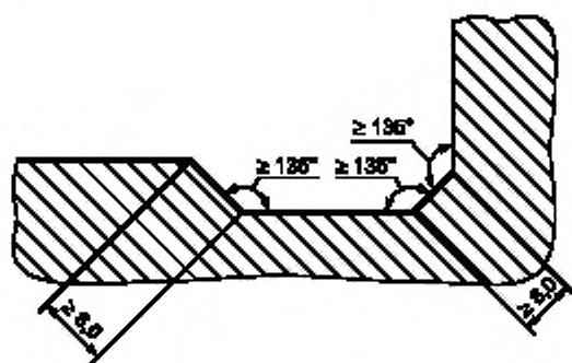
Рисунок A.3 — Углы в пищевой зоне
