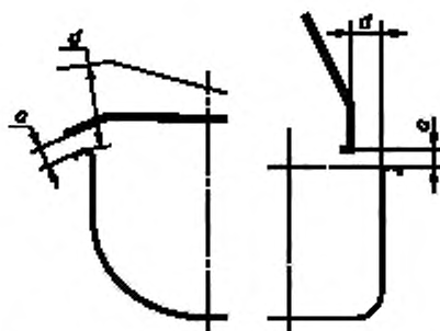
a — расстояние между защитным устройством дежи и ободом вращающейся дежи; d — расстояние между верхним ободом дежи и положением внешней кромки защитного устройства, когда блокировочное устройство работает
