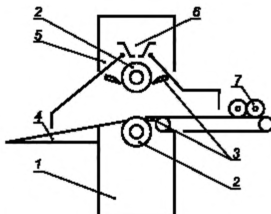
1 — привод валов (электромотор). 2 — валы. 3 — устройства для удаления остатков теста с валов. 4 — стол или транспортер. 5 — управляющая система. 6 — узел для посыпания муки. 7 — устройства для нарезки и закатывания теста
