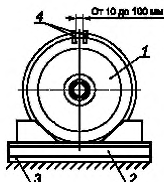
Рисунок А.1 — Схема установки колесной пары
