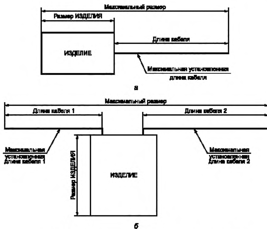
Рисунок ААА.2 — Примеры определения максимальных размеров ИЗДЕЛИЙ с одним (а) и двумя (б) кабелями [см. 36.202.6 перечисления а) 5 и б)]
