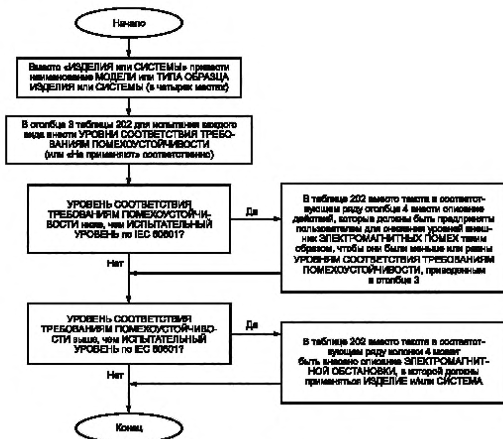
Рисунок 203 — Порядок заполнения таблицы 202 [см. 6.8.3.201, перечисление а) 6)]
