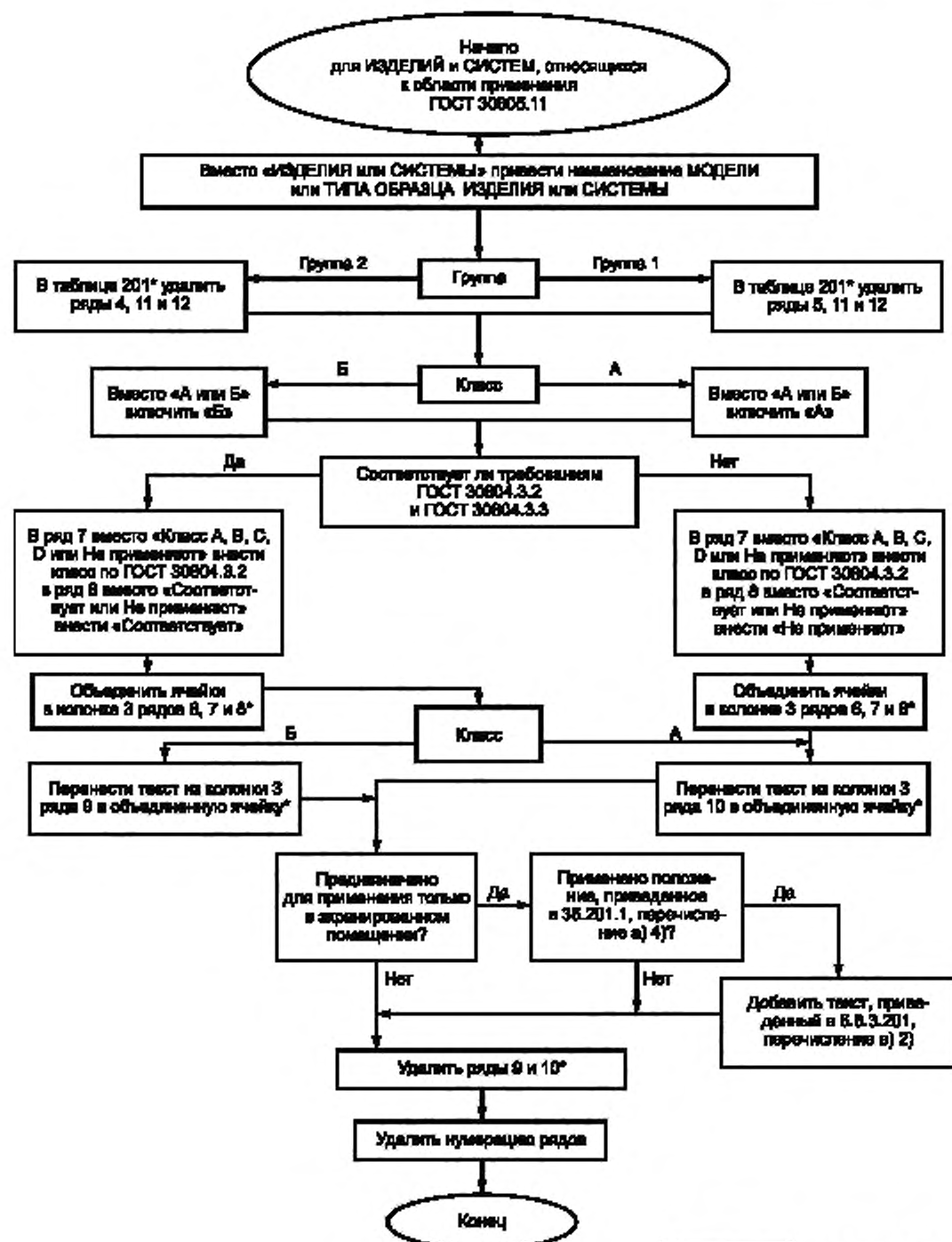
Рисунок 201 — Порядок заполнения таблицы 201 для ИЗДЕЛИЙ и СИСТЕМ, относящихся к области применения ГОСТ 30805.11 [см. 6.8.3.201, перечисление а) 3)]
