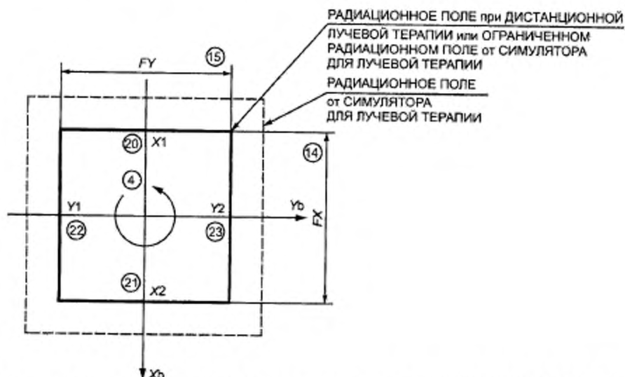
Рисунок 103 – Движения ИЗДЕЛИЯ и шкалы. Вид РАДИАЦИОННОГО ПОЛЯ при ДИСТАНЦИОННОЙ ЛУЧЕВОЙ ТЕРАПИИ или ОГРАНИЧЕННОМ РАДИАЦИОННОМ ПОЛЕ на СИМУЛЯТОРЕ ДЛЯ ЛУЧЕВОЙ ТЕРАПИИ относительно ИСТОЧНИКА ИЗЛУЧЕНИЯ (см. ниже таблицу).
