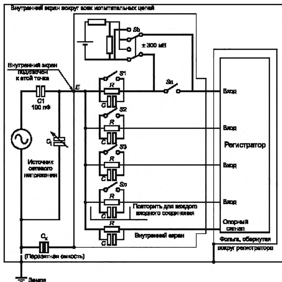
Рисунок 105 — Цепь для испытания подавления синфазной помехи (51.5.3)
