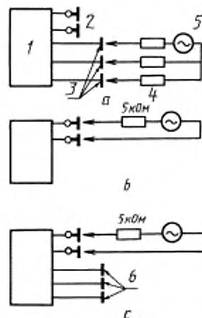
1 — АППАРАТ; 2 — ЭЛЕКТРОДЫ ДЕФИБРИЛЛЯТОРА разомкнуты; 3 — электроды монитора; 4 — резисторы сопротивлением 25 кОм; 5 — генератор с изолированным выходом, формирующий синусоидальный сигнал частотой 10 Гц «пик-провал» 1 мВ; 6 — электроды монитора подсоединены к АППАРАТУ, но разомкнуты
