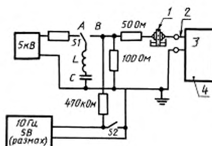
1 — электроды аппарата на губке, насыщенной раствором; 2 — соединительный кабель аппарата; 3 — отдельный вход монитора; 4 — ДЕФИБРИЛЛЯТОР-МОНИТОР
