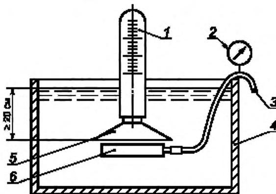
1 — градуированный цилиндрический сосуд (8.2.3); 2 — манометр для измерения испытательного давления; 3 — газопровод; 4 — водяная ванна (8.2.1); 5 — воронка (8.2.4); 6 — испытуемое устройство
