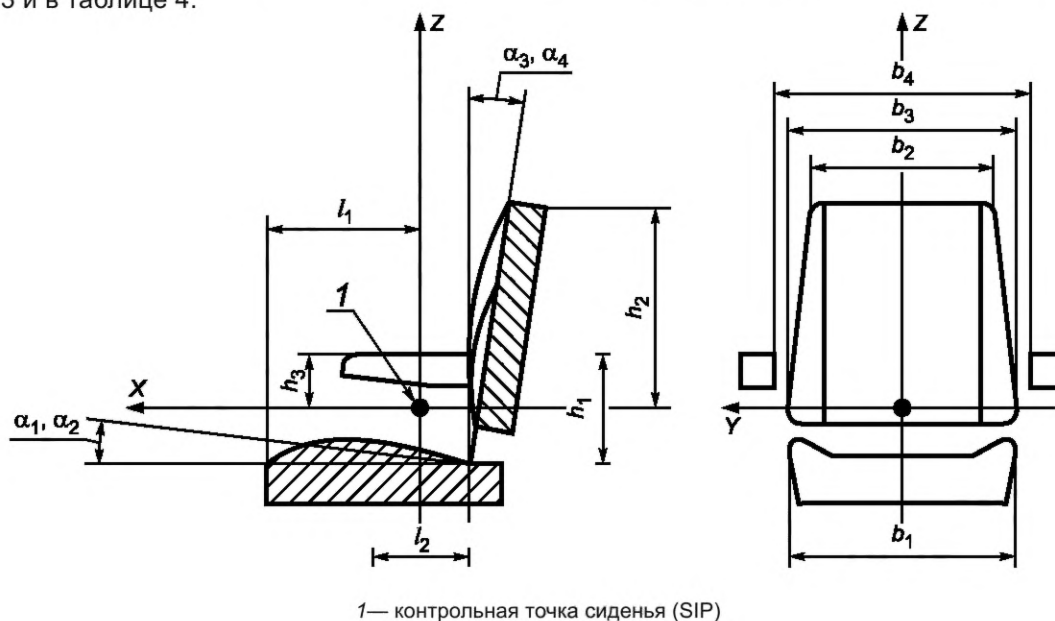
Рисунок 3 — Сиденье оператора
