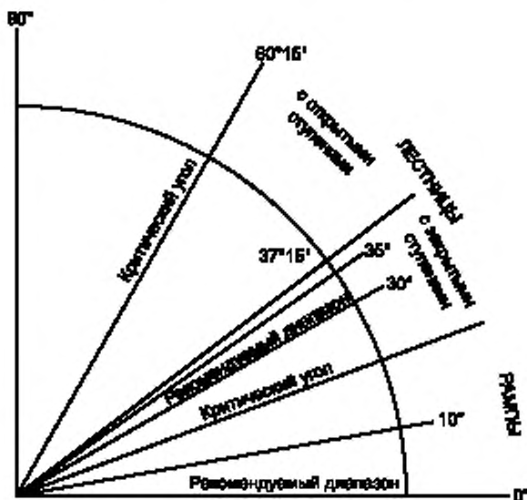
Рисунок 1 — Углы наклона средств доступа к рабочему месту
