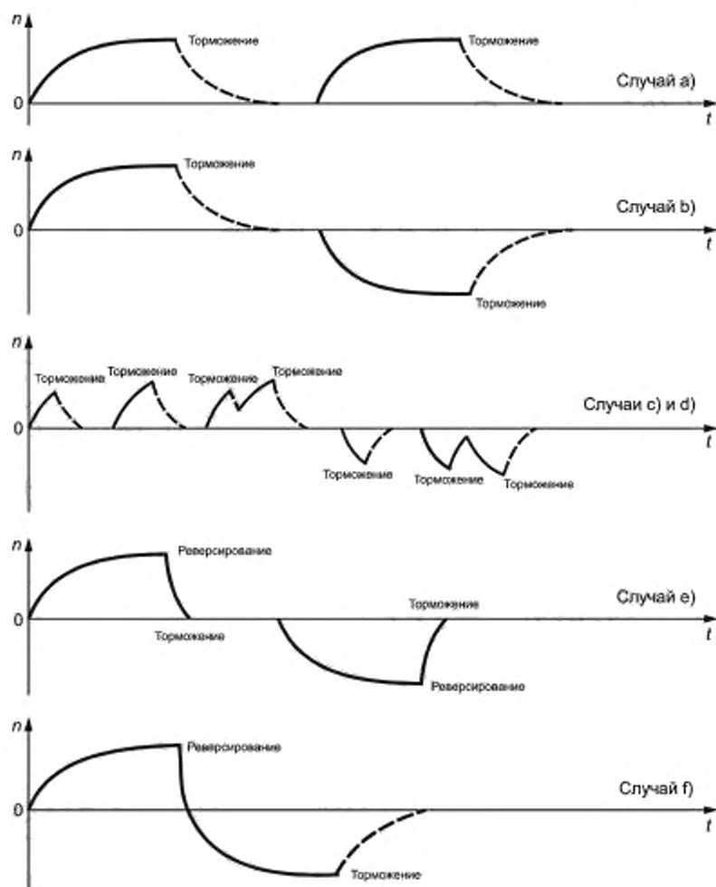
Рисунок С.6 — Примеры кривых скорости/времени для случаев а)–f) по 5.3.5.6.1
