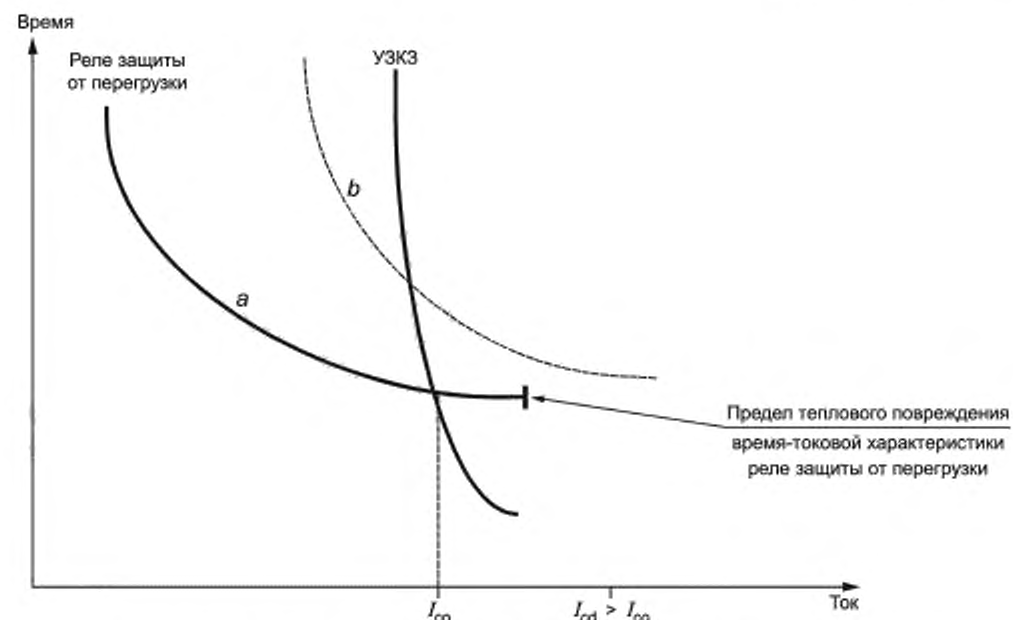
а) Координация с плавким предохранителем
