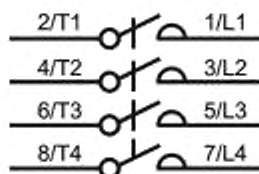
Рисунок А.1 — Клеммы главных цепей
