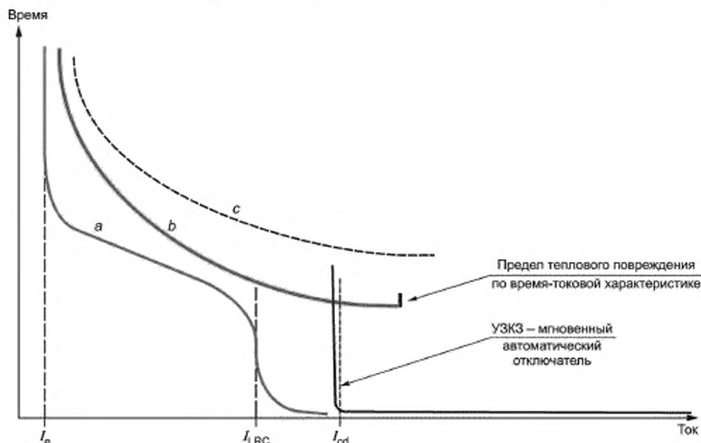
a — ток пуска двигателя; b — средняя время-токовая характеристика реле перегрузки в холодном состоянии; c — выдерживаемая время-токовая характеристика контактора по 9.3.5
