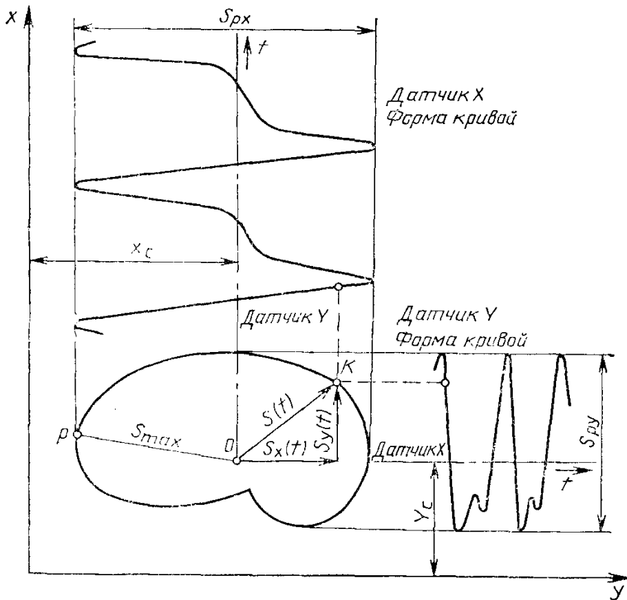
Траектория виброперемещения контролируемого сечения ротора
