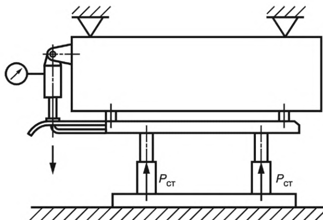
Рисунок А.1 — Схема нагружения передней консоли перекрытия
