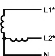
Рисунок 2 – Однофазная трехпроводная электрическая цепь
