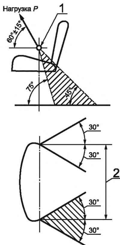
1 — контрольная точка сиденья по ГОСТ 27715; 2 — ширина подушки
