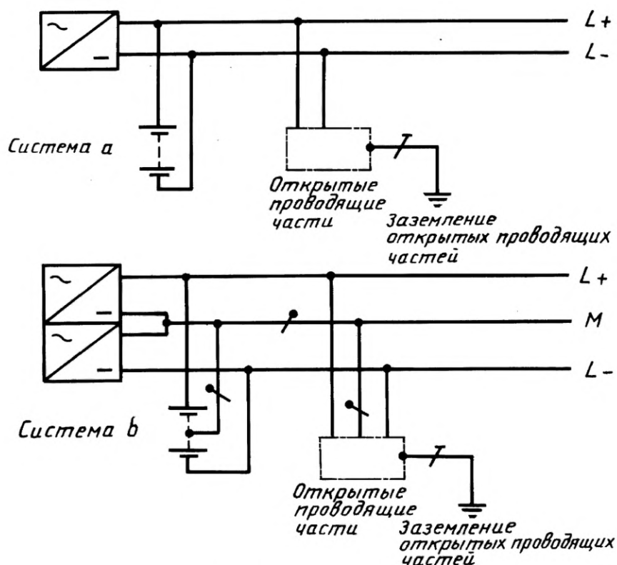
Рисунок 31К — Система ИТ постоянного тока
