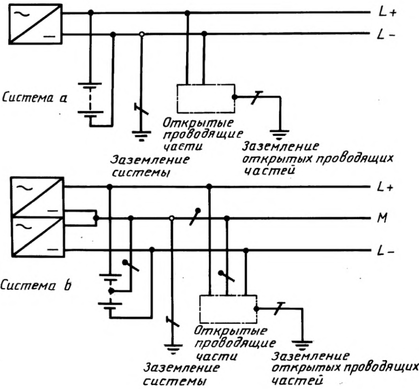
Рисунок 31J — Система ТТ постоянного тока
