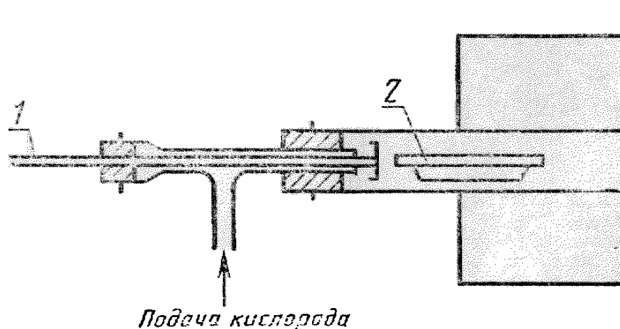
1 — толкатель; 2 — лодочка
