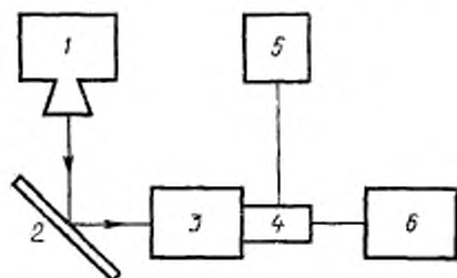
Блок-схема установки для измерения спектрального состава излучения экранов
