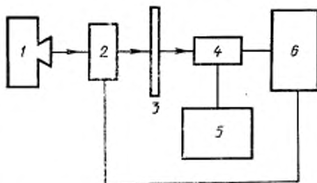
Блок-схема установки для измерения послесвечения экранов
