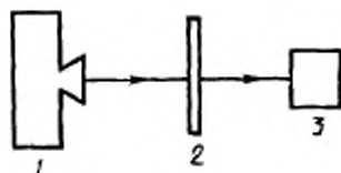
Блок-схема установки для измерения яркости свечения экранов
