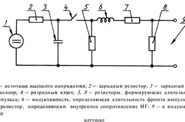
Рисунок 3 — Схема ИГ
