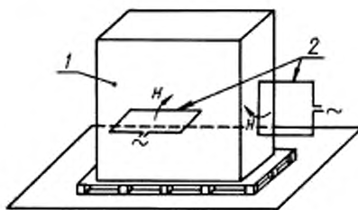
1 — ИТС; 2 — индукционная катушка
