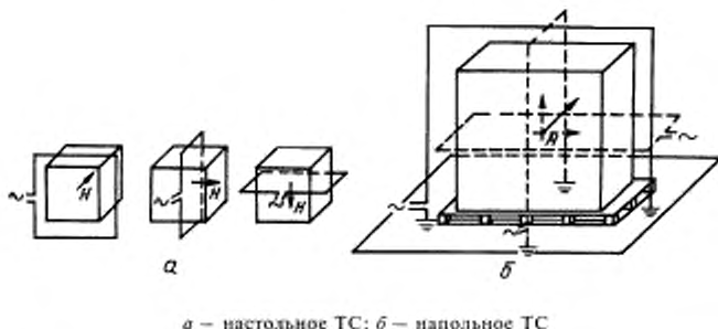
Рисунок 1 — Схема воздействия ИМП на ТС с использованием иммерсионного метода
