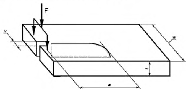
a – Схема испытания
