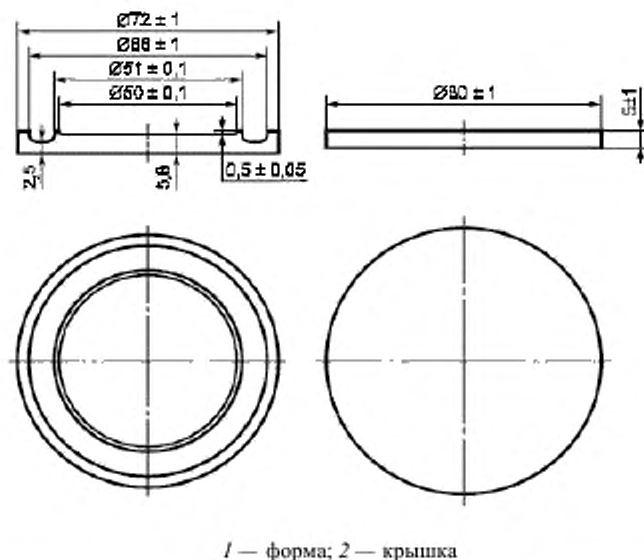
Рисунок 2 — Форма из нержавеющей стали и крышка для испытаний на цветостойкость, водопоглощение и растворимость
