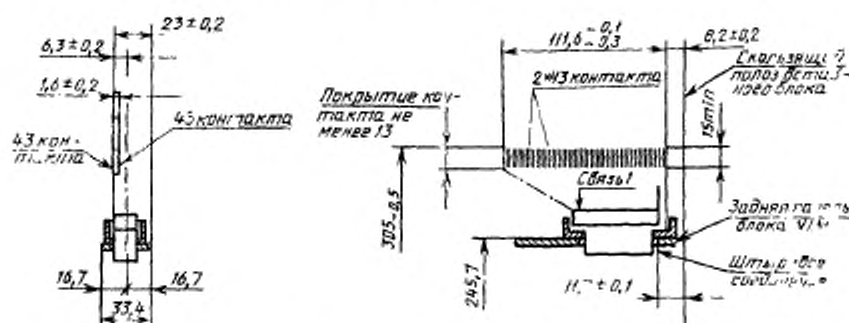
Рисунок 6 — Вентилируемый крейт. Вид спереди
