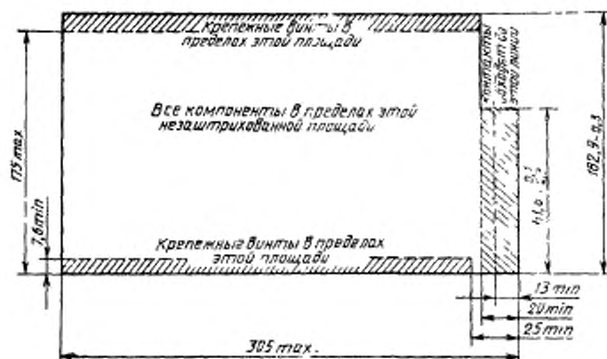
Рисунок 8 — Типовая печатная плата
