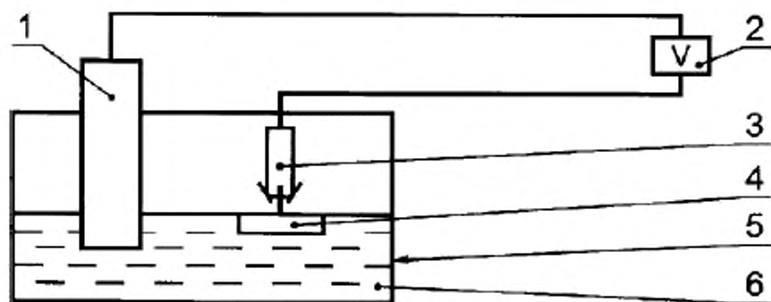
1 — стандартный электрод (хлорсеребряный ЭВЛ-1МЗ или платиновый ЭТПЛ-01М); 2 — высокоомный вольтметр с погрешностью измерения \pm 10\% ; 3 — зажим типа «крокодиль»; 4 — протезы с покрытием; 5 — стеклянный стакан или электрохимическая ванночка; 6 — модельная среда (см. 5.6.1)
