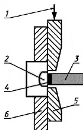
1 — нагрузка; 2 — субстрат — фрагмент зуба в монтажном блоке с открытой для испытания поверхностью эмали; 3 — испытываемый восстановительный материал; 4 — адгезив; 5 — нагружающая пластина в приспособлении для сдвига; 6 — кольцо в приспособлении для сдвига
