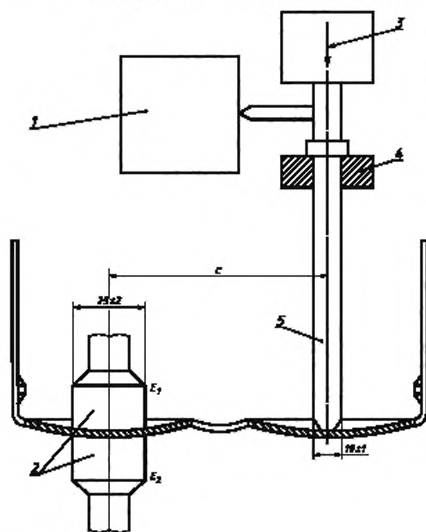
Рисунок А.1 — Схема испытательной установки
