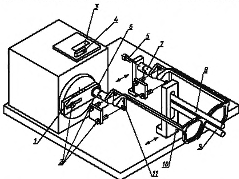
1 — шкала амплитуды смещения оправы; 2 — крепежные винты; 3 — окно счетчика; 4 — контрольный выключатель; 5 — фиксирующий винт; 6 — шариковый подшипник; 7 — универсальный шарнир; 8 — регулируемый ограничитель моста; 9 — регулируемый узел поддержки моста; 10 — регулируемая стойка для различных размеров очковых оправ; 11 — подвижный зажим
