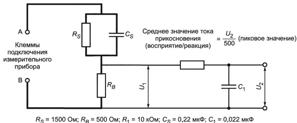
Рисунок N.2 — Измерительный прибор
