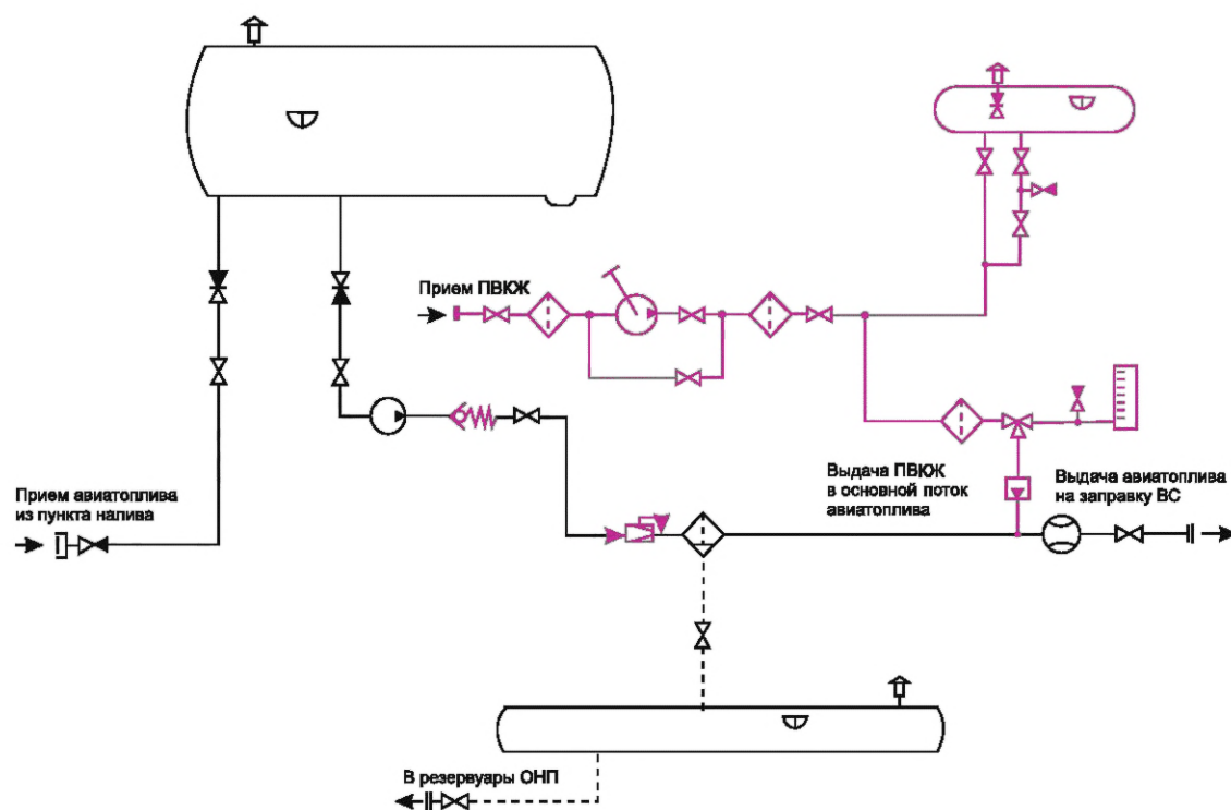
Рисунок Б.8 — ТМ АТО заправки ВС из собственной цистерны с возможностью ввода ПВКЖ
