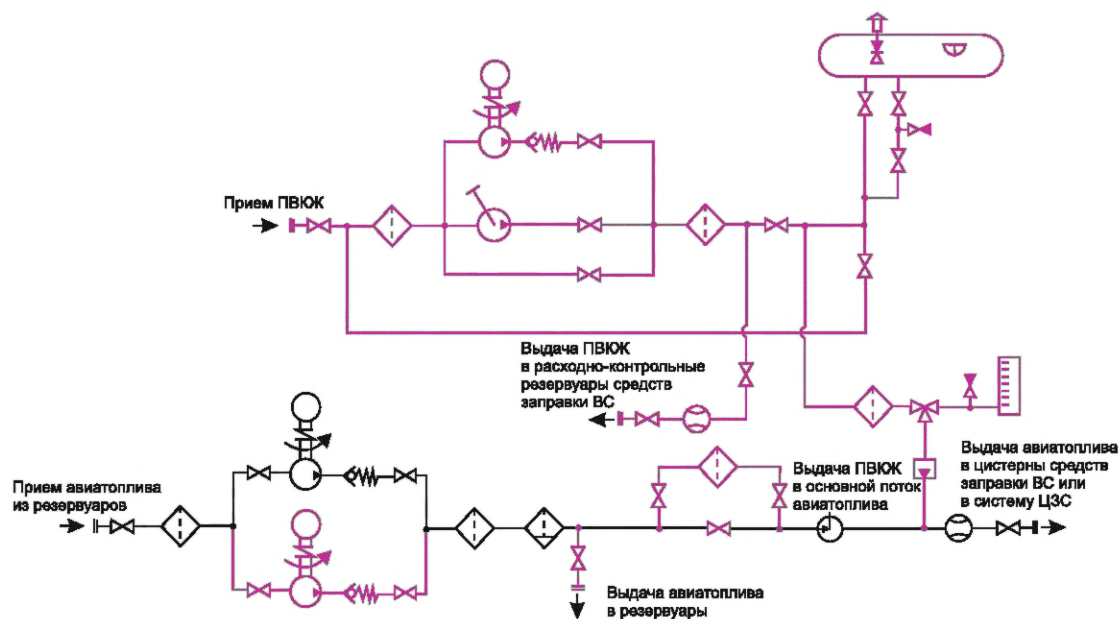
Рисунок Б.4 — ТМ АТО выдачи авиатоплива из резервуаров расходных в систему ЦЗС, на пункты налива средств заправки ВС, в цистерны средств заправки ВС, приема и выдачи ПВКЖ в резервуары расходно-контрольных средств заправки ВС и внутрискладской перекачки авиатоплива
