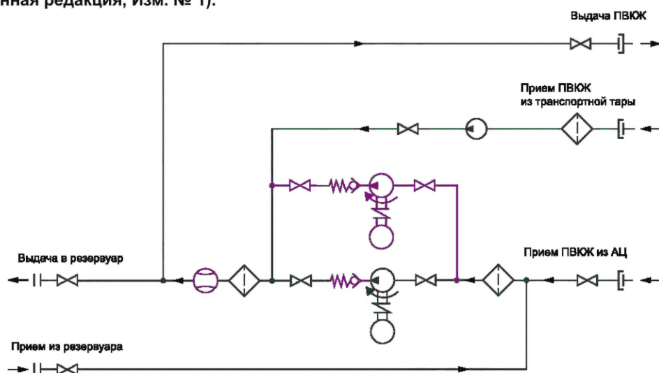
Рисунок Б.9 — ТМ АТО приема, внутрискладских перекачек и выдачи ПВКЖ
