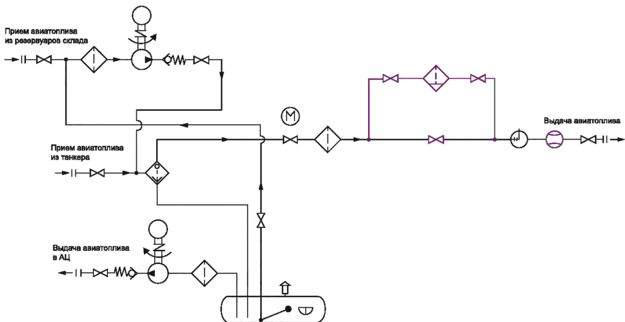
Рисунок Б.3 — ТМ АТО приема авиатоплива из танков нефтепродуктовых судов, стоящих на рейде, с гидроопорожнением шлангующих устройств, внутрискладских перекачек
