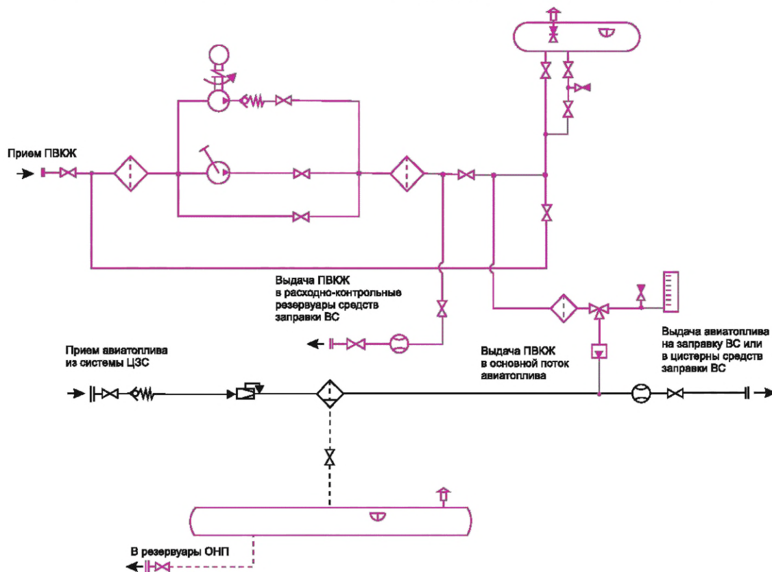
Рисунок Б.5 — ТМ АТО заправки ВС из системы ЦЗС с возможностью ввода ПВКЖ, выдачи авиатоплива в чистом виде из системы ЦЗС в цистерны средств заправки ВС
