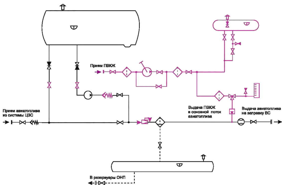
Рисунок Б.7 — ТМ АТО заправки ВС из системы ЦЗС или из собственной цистерны с возможностью ввода ПВКЖ и функцией наполнения цистерны из системы ЦЗС
