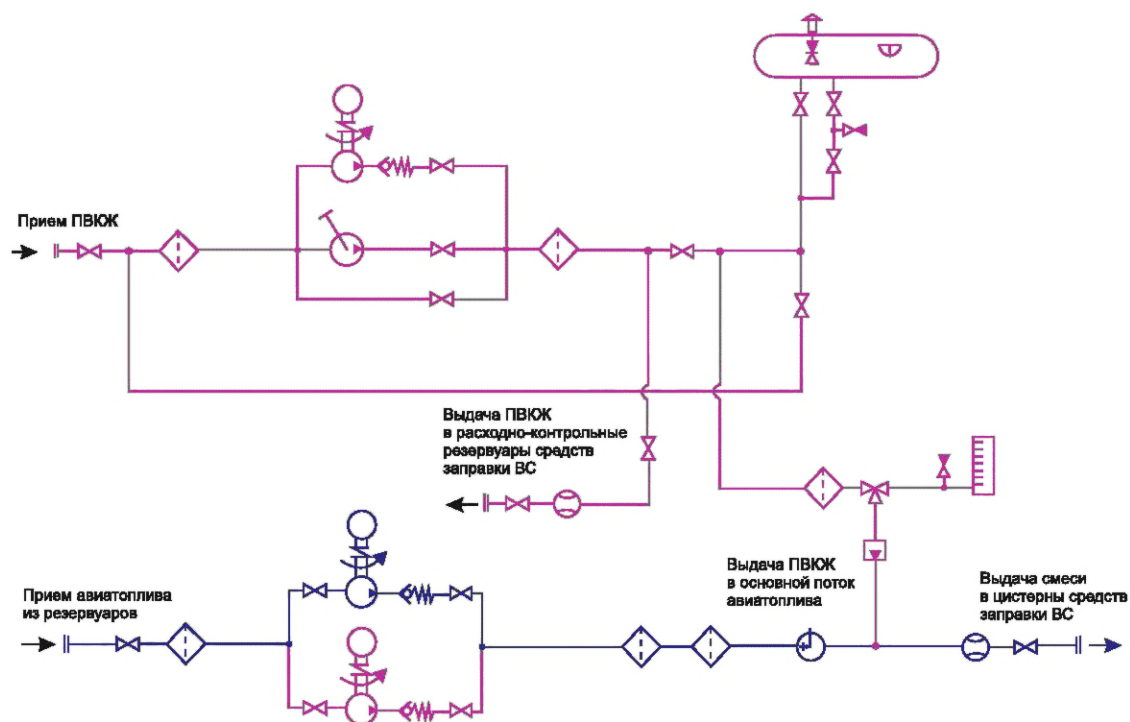
Рисунок Б.12 — ТМ АТО выдачи смеси из резервуаров расходных в средства заправки ВС с возможностью ввода ПВКЖ, приема и выдачи ПВКЖ в резервуары расходно-контрольные средств заправки ВС
