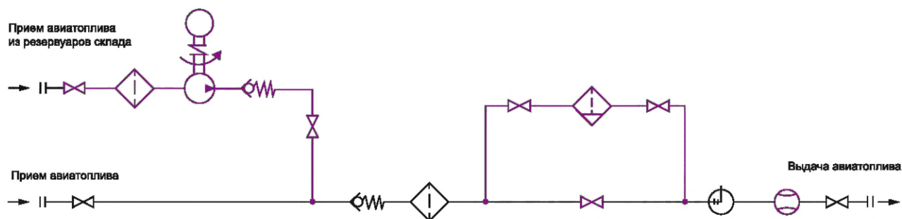
Рисунок Б.2 — ТМ АТО приема авиатоплива из магистрального трубопровода, танков пришвартованных нефтепродуктовых судов и нефтепродуктовых судов, стоящих на рейде, с пневмоопорожнением шлангующих устройств, внутрискладских перекачек
