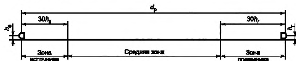
Рисунок 1 — Три основные зоны при определении затухания из-за влияния земли
