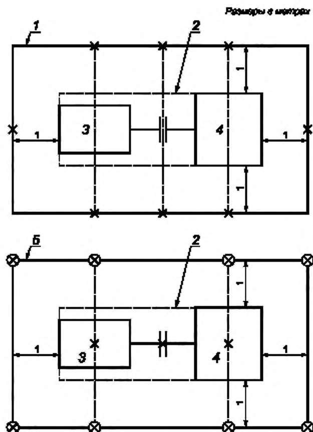
1 — медианная плоскость измерительной поверхности; 2 — огибающий параллелепипед; 3 — привод, 4 — насос; 5 — верхняя грань измерительной поверхности x — положения микрофонов для ориентировочного метода; x и o — положения микрофонов для технического метода
