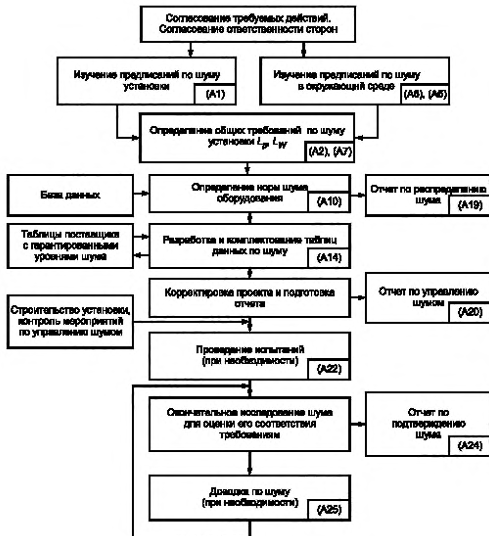
Рисунок А.1 — Схема управления шумом
