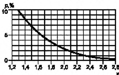
Рисунок 1 — Проценти́лы p максимальных уровней звукового давления единичных звуковых событий, превышающих на y стандартных отклонений среднеарифметическое значение при нормальном распределении максимальных уровней звукового давления
