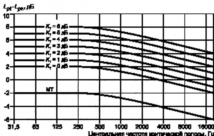
Рисунок С.1 — Маскирующий порог слышимости (МТ) и графики для определения коррекции K_T
