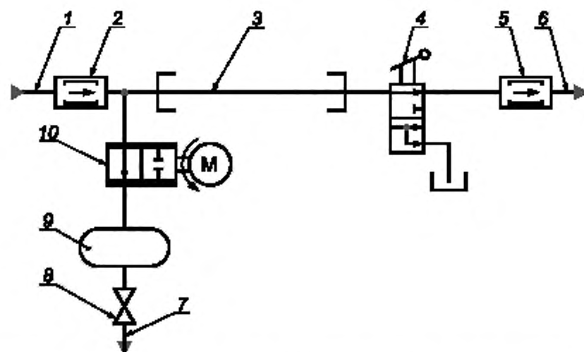
1 — магистраль нагнетания жидкости от насосной станции; 2, 5 — гаситель колебаний давления жидкости; 3 — очищаемая магистраль трубопровода; 4 — прободоотборник; 6, 7 — магистраль слива в насосную станцию; 8 — регулирующий вентиль; 9 — баллон блока акустической развязки; 10 — генератор колебаний жидкости
