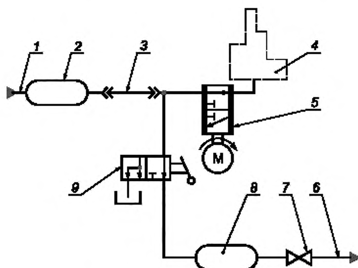
Рисунок 4 — Схема пульты для гидродинамической очистки проточных агрегатов
