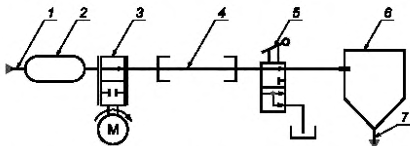
1 — магистраль нагнетания жидкости от насосной станции; 2 — баллон блока акустической развязки; 3 — генератор колебаний жидкости; 4 — очищаемый трубопровод; 5 — прободоотборник; 6 — сливная емкость; 7 — магистраль слива в насосную станцию
