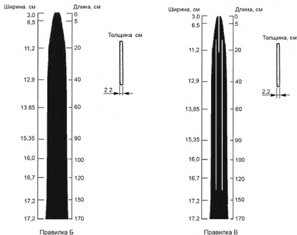
Рисунок 2 — Правилки Б и В
