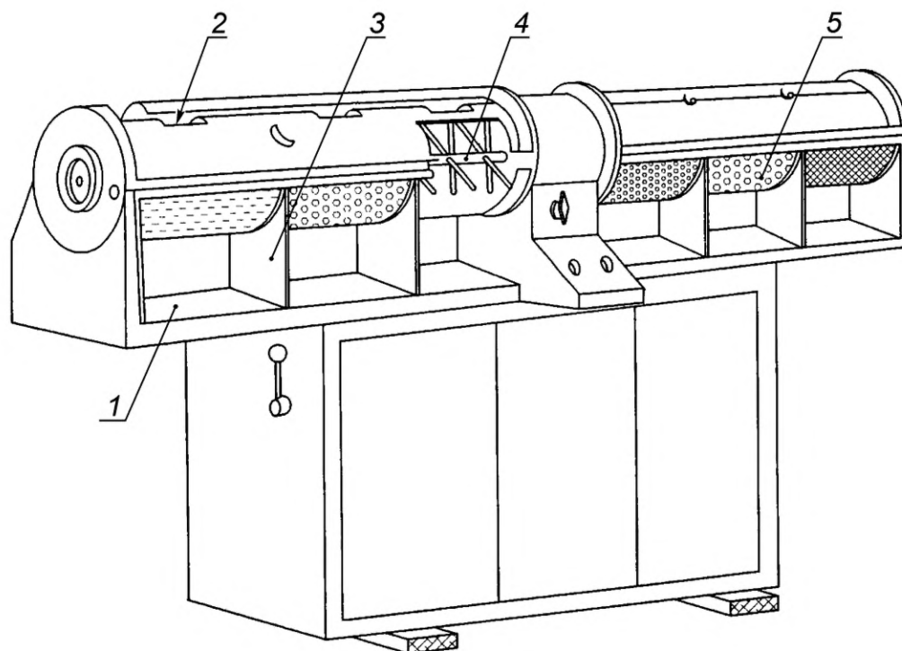
1 — рабочая камера; 2 — загрузочная воронка; 3 — перегородка; 4 — вал с колodkaми; 5 — сито
