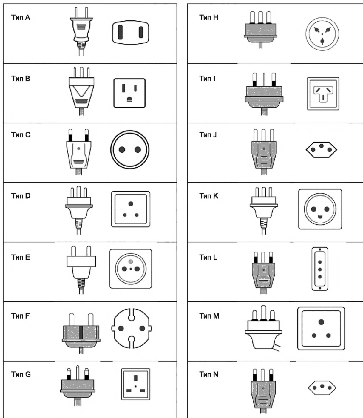
Рисунок АА.1 — Типы вилок разных стран
