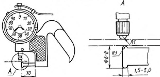
Прибор с круговой шкалой
