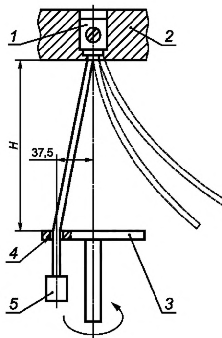
1 — зажим; 2 — неподвижная часть; 3 — пластина; 4 — втулка; 5 — груз
