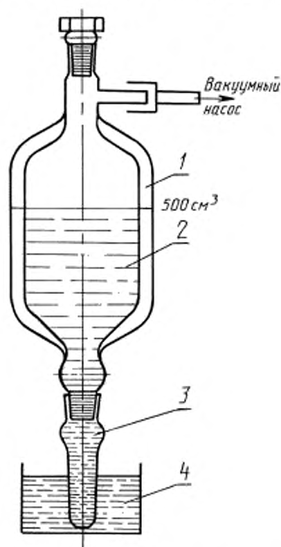
1 — стекланный сосуд с двойными стенками (п. 4.1) с нижним шлифом и градуировочной линией; 2 — заданная проба, 3 — съемный элемент со шлифом; 4 — нагревательное устройство
