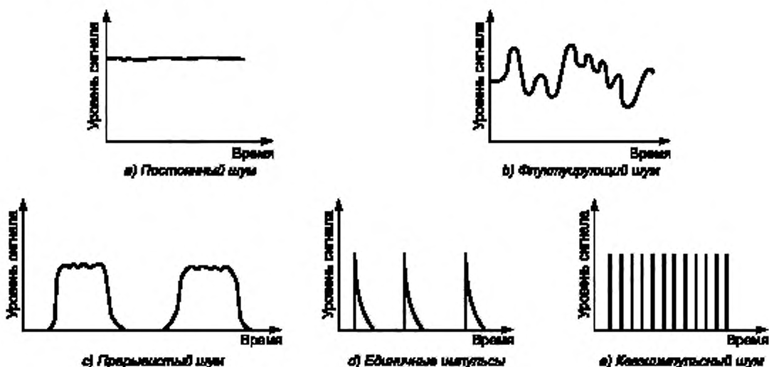
Рисунок Е.1 — Примеры шума различного вида
