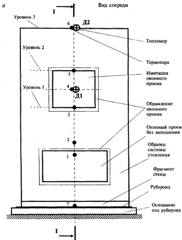
Рисунок 2 — Схема установки с образцом системы утепления
