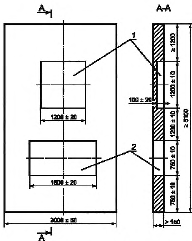
Рисунок 1 — Фрагмент стены
