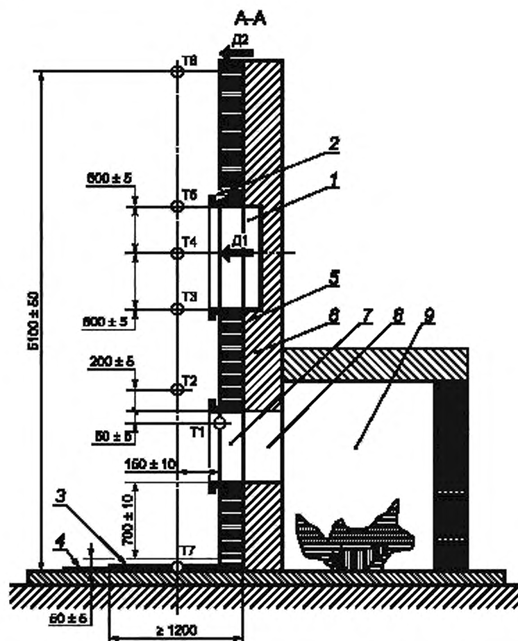
Т1 — Т7 — термопары; Д1, Д2 — тепломеры; 1 — имитация оконного проема; 2 — обрамление оконного проема (если предусматривается); 3 — рубероид; 4 — основание под рубероид; 5 — образец теплоизоляции, отделки или облицовки; 6 — фрагмент стены; 7 — оконный проем без заполнения в испытуемой конструкции; 8 — открытый проем фрагмента стены; 9 — огневая камера
