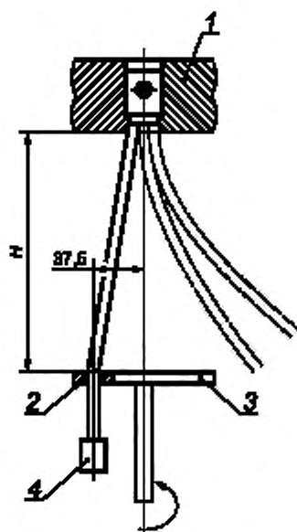
1 — узел фиксации; 2 — гильза; 3 — диск; 4 — груз
