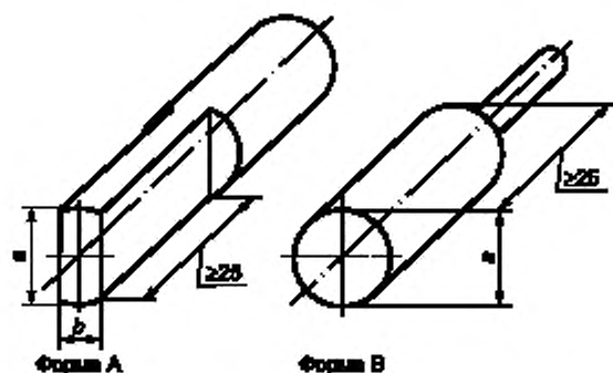
Рисунок 2 — Шулы формы А и В (см. 8.2.4.5.2 и таблицу 7)
