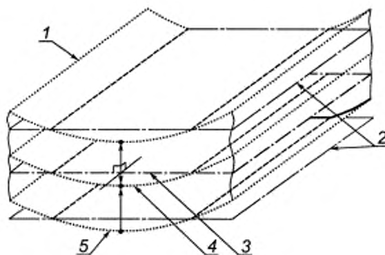
1 — выявленная поверхность; 2 — присоединенная плоскость; 3 — присоединенная плоскость симметрии; 4 — выявленная средняя поверхность; 5 — выявленная поверхность
