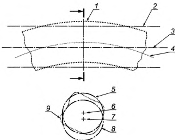
1 — выявленная поверхность; 2 — присоединенный цилиндр; 3 — ось присоединенного цилиндра; 4 — выявленная средняя линия; 5 — присоединенная окружность; 6 — центр присоединенной окружности; 7 — ось присоединенного цилиндра; 8 — присоединенный цилиндр; 9 — выявленная линия
