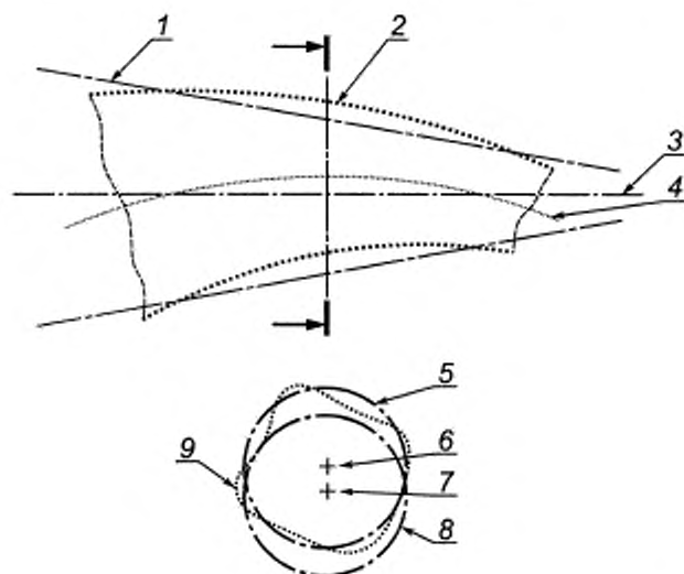
1 — присоединенный конус; 2 — выявленная поверхность; 3 — ось присоединенного конуса; 4 — выявленная средняя линия; 5 — присоединенная окружность; 6 — центр присоединенной окружности; 7 — ось присоединенного конуса; 8 — присоединенный конус; 9 — выявленная линия
