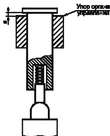
Рисунок 3 — Разность в между остаточным ходом органа управления и контактного элемента
