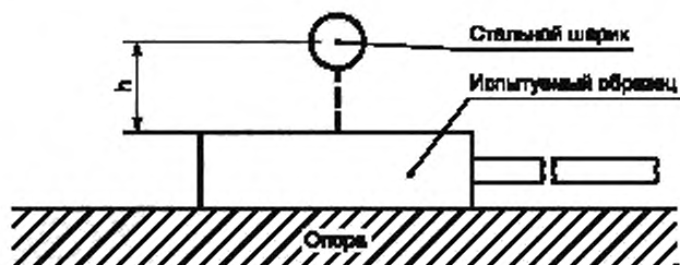
Рисунок Ф.2 — Испытательная установка
