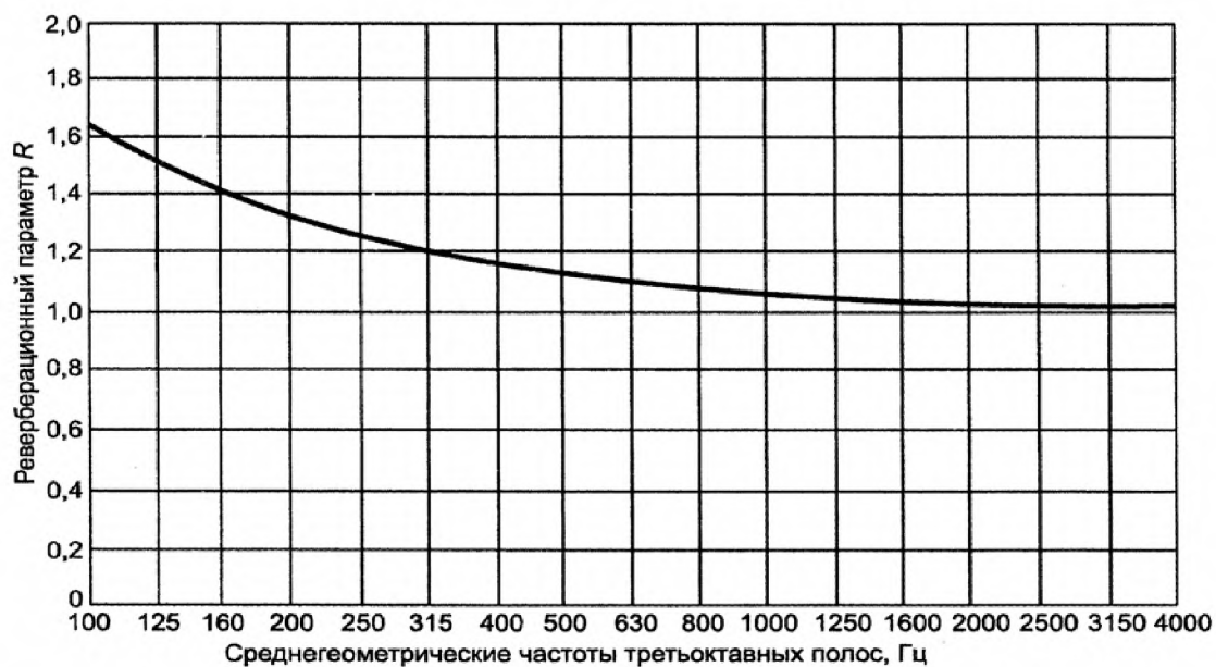
Рисунок Б.3 – Значение реверберационного параметра R для камеры объемом 70 \text{ м}^3 в функции среднегеометрической частоты третьооктавной полосы
