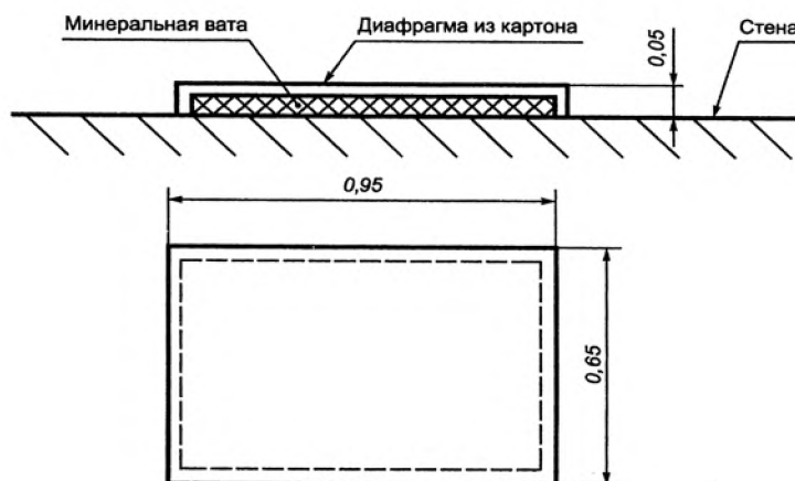
Рисунок Б.1 – Резонансный поглотитель с диафрагмой из картона
