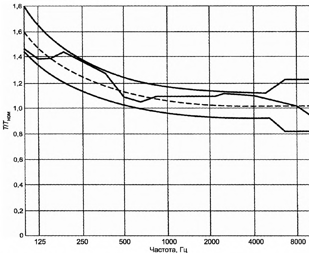
Рисунок Б.4 – Предельные кривые для отношения времени реверберации T к номинальному времени реверберации T_{\text{ном}} для камеры объемом 70 \text{ м}^3
