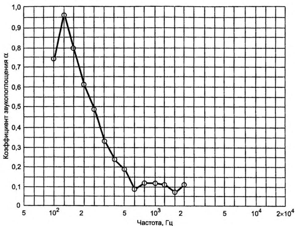
Рисунок Б.1 – Резонансный поглотитель с диафрагмой из картона
