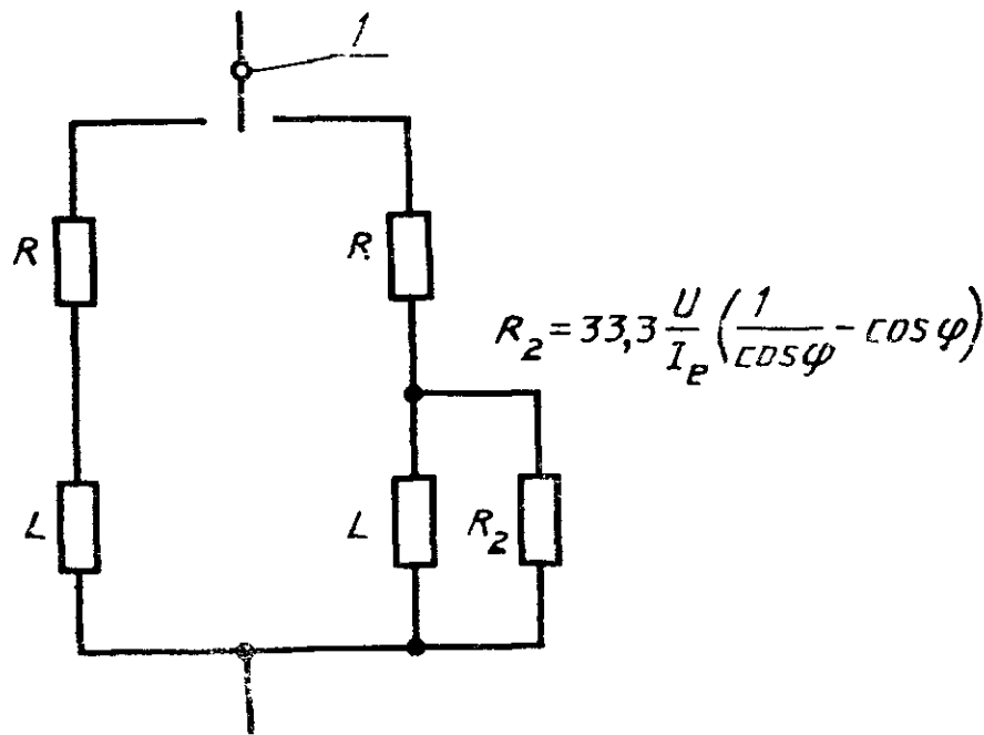
Испытательная схема (см. 8.3.3.5 гл. 1)
