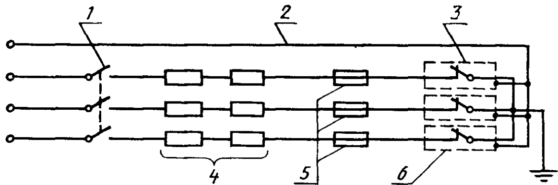
Испытательная схема (см. 8.3.4.2 гл. 1)
