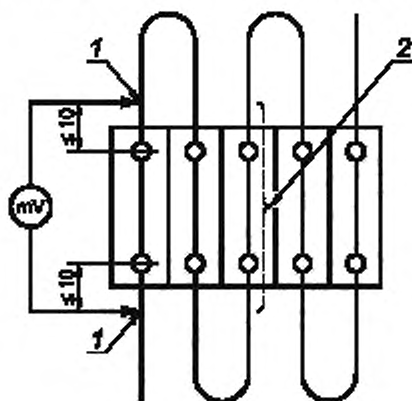
1 — место измерения падения напряжения мультиметром; 2 — место измерения температуры
